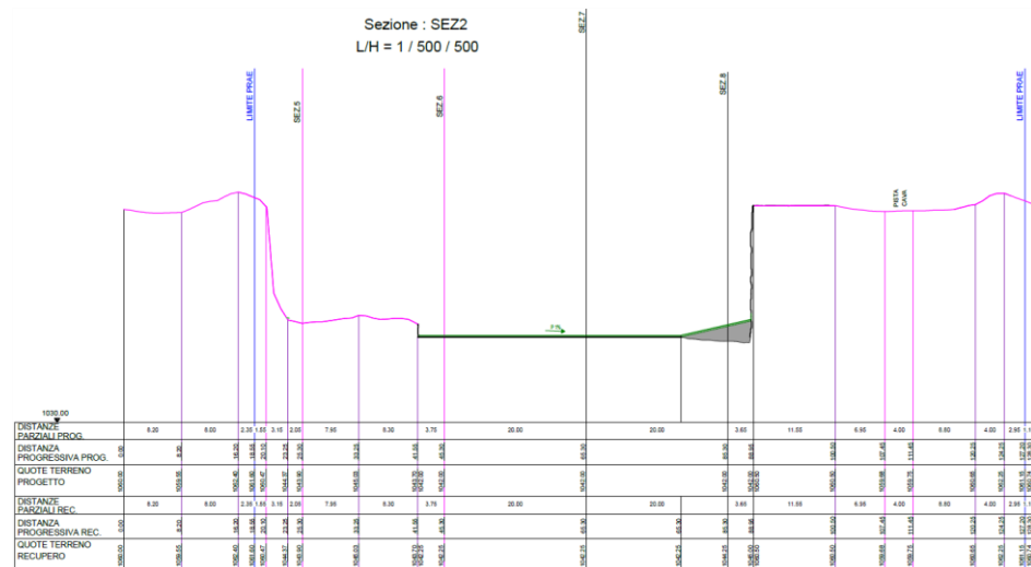
Sezioni tipo di recupero
