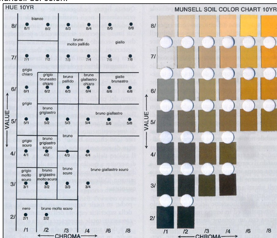
La tavola delle Munsell Soil Color Charts 10YR
